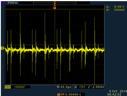
Fig.2 Misura su una porta Ethernet con inverter in funzione senza filtro EMI-RFI
